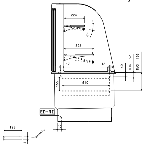
Zij aanzicht
